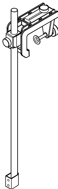
万能パイプ取付金具 (BP10)
