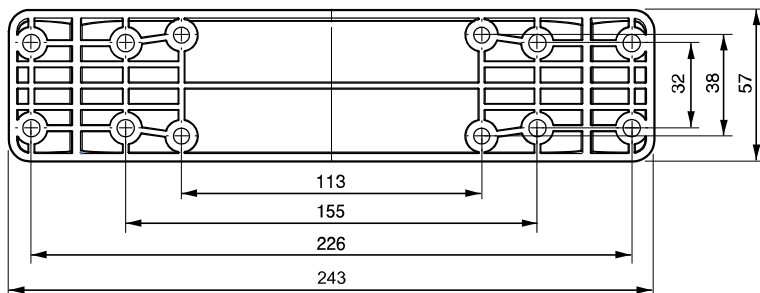
〈架台取付け穴寸法図〉
