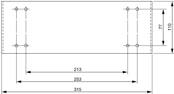
〈架台取付け穴寸法図〉
